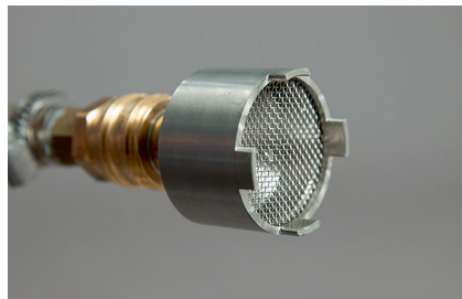
Sugsystem med filter
